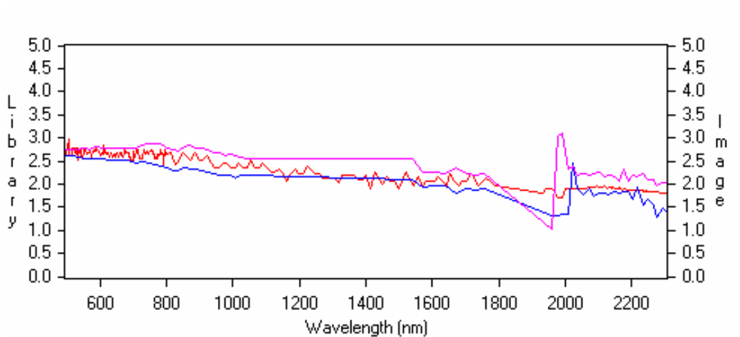
Rys. 35. Krzywe spektralne wody po kalibracji radiometrycznej metodą Empiric Line na obrazach wstępnie przetworzonych za pomocą metody MNF (powiększenie), (czerwona – wzorzec JPL, niebieska bez transformacji MNF, fioletowa z uwzględnieniem transformacji MNF)
