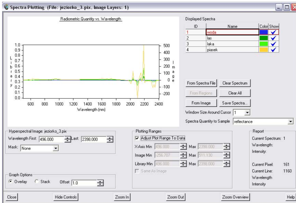
Rys. 45. Krzywe spektralne przed korekcją radiometryczną (niebieska – woda, ciemnozielona – las, jasnozielona – łąka, żółta – piasek)
