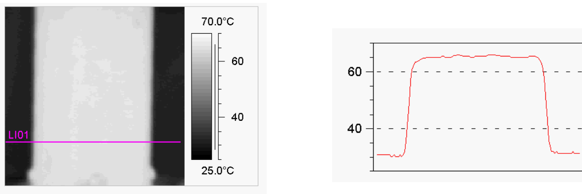
Rys 1. Zniekształcenie obrazu temperatury na termogramie powierzchni walcowej
