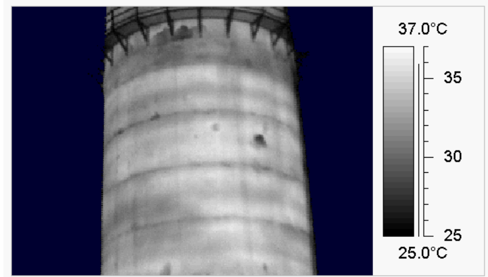
Rys 2. Geometryczne zniekształcenia termograficznego obrazu komina.
