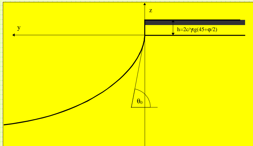
Schemat obliczeniowy do metody Sokółowskiego-Senkowa
