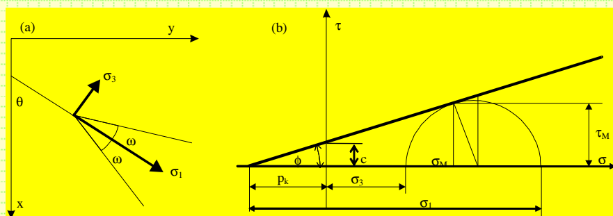
Ilustracja graficzna założeń teorii stanów granicznych
