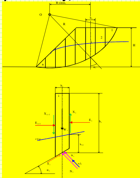
Schemat obliczeniowy metody Bishopa
