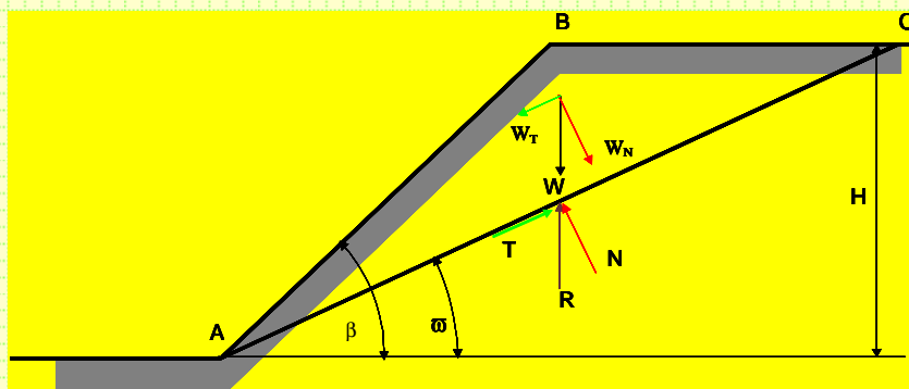
Schemat obliczeniowy metody Cullmana
