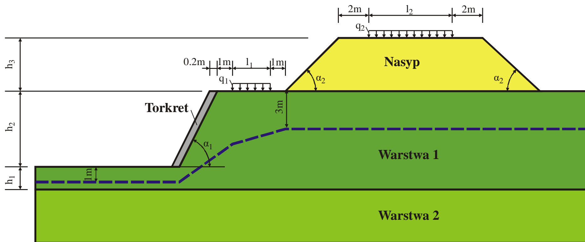
Rys. 1. Geometria modelu.
