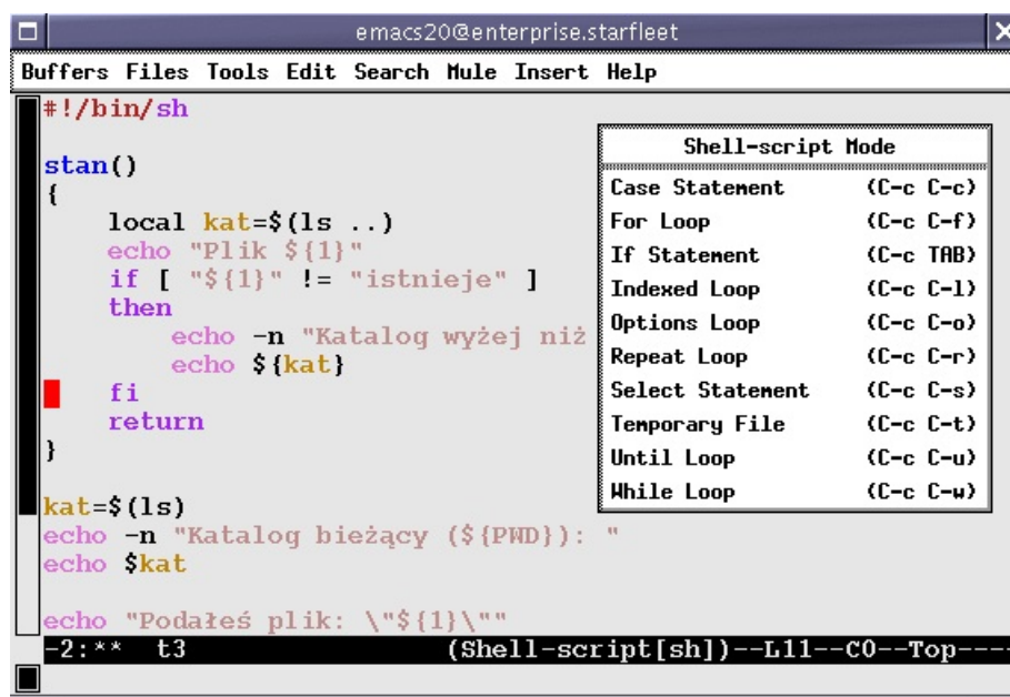
Rysunek 1: Tryb sh GNU Emacsa
