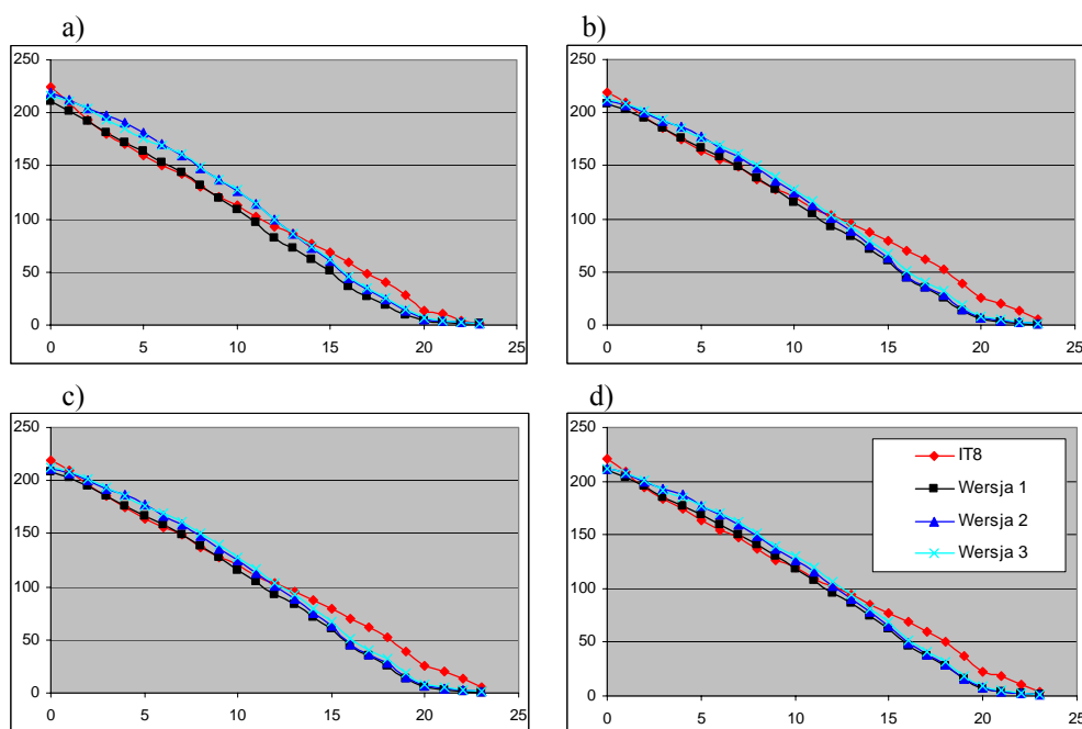
Rys. 4. a) kanał R; b) kanał G; c) kanał B; d) średnia jasność RGB. Przenoszenie gęstości optycznej. Oś x – pola klina szarości. Oś y – średnie wartości jasności pikseli.
