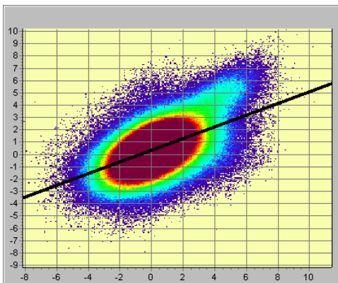
Figure 5. Regress analyze, ERS99\_97=0.49 ERS96\_97+0.34 , r=0.52
