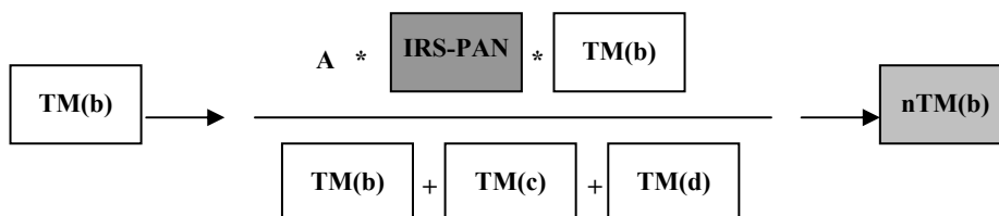
Rys. 4. Integracja danych metodami: transformacji Brovey’ a ( A=1 ), CN ( A=3 ), Wiemkera ( A obliczane każdorazowo dla konkretnego kanału)
