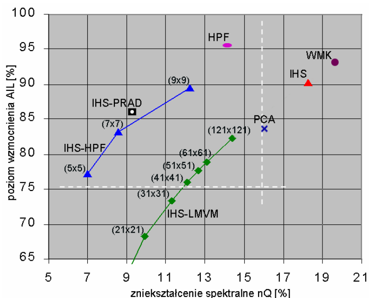
Rys. 8. Diagram wyników: Ocena formalna grupy metod IHS na tle metod HPF, PCA, WMK. Liczby oznaczają wielkość okna obliczeń. Wartości średnie dla 6. kanałów.
