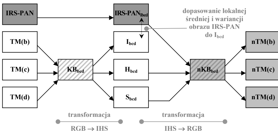
Rys. 7. Integracja danych metodą IHS-LMVM.
