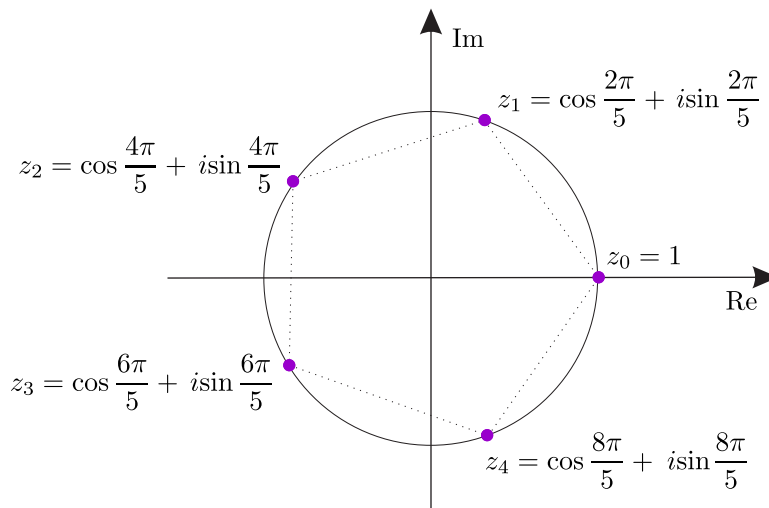
Wykres 2. Interpretacja geometryczna rozwiązań równania z^5 = 1 .
