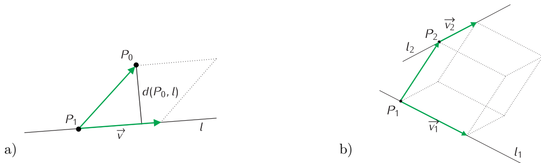
Wykres 7. Odległość punktu P_0 od prostej l (rys. a) oraz odległość między prostymi skośnymi l_1 i l_2 (rys. b).
