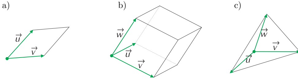
Wykres 6. Zastosowanie iloczynów wektorów: a) wektorowego; b) i c) mieszanego
