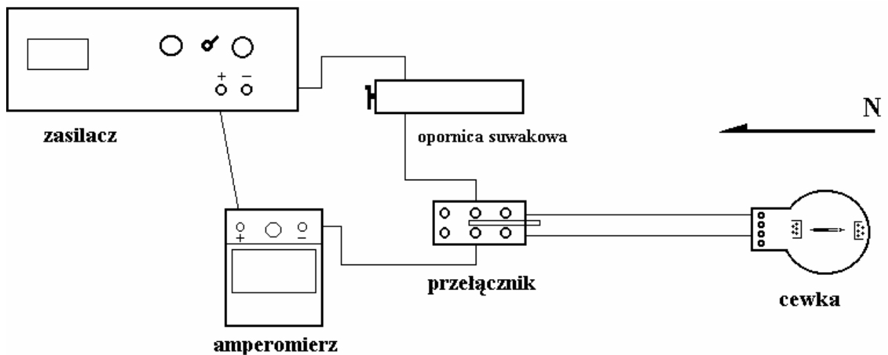
Rys. w1. Układ elektryczny busoli stycznych.
