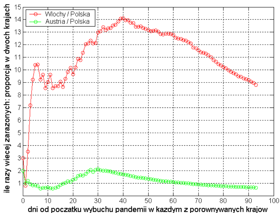
Rys. 7. Proporcja zarażonych (według oficjalnych danych) w kolejnych dniach od wybuchu pandemii – czyli przykładowo: ostatni wynik dotyczy danych z Polski z dnia 6 czerwca, natomiast z Włoch z 22 maja, a dla Austrii z 29 maja, ponieważ to był 88. dzień pandemii w tych krajach (według przyjętego tu kryterium).
