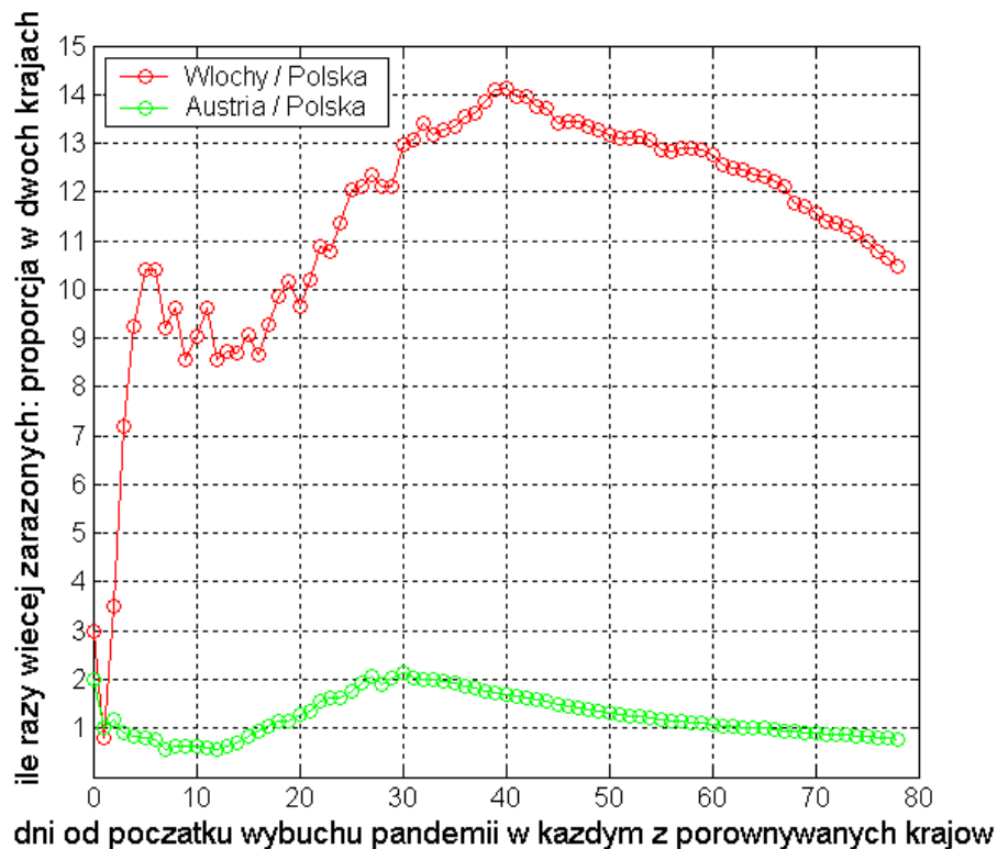
Rys. 7. Proporcja zarażonych (według oficjalnych danych) w kolejnych dniach od wybuchu pandemii – czyli przykładowo: ostatni wynik dotyczy danych z Polski z dnia 22 maja, natomiast z Włoch z 7 maja, a dla Austrii z 14 maja, ponieważ to był 78. dzień pandemii w tych krajach (według przyjętego tu kryterium).
