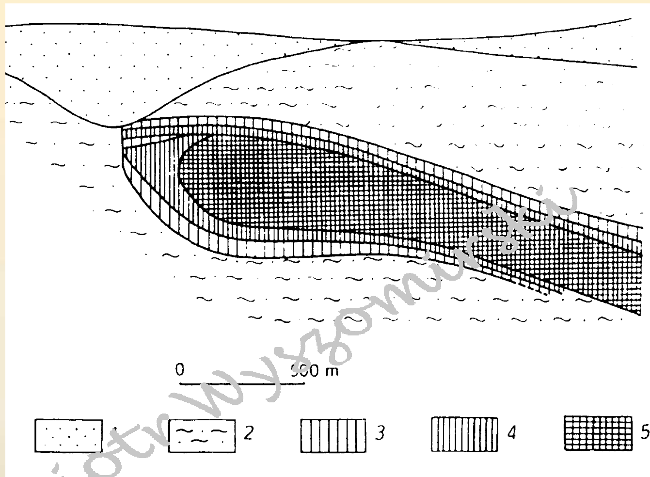
Rys.7. Przekrój przez złożę anhydrytu i gipsu Nowy Łąd w Niwnicach k. Lwówka Śląskiego (W.Narębski 1959).
