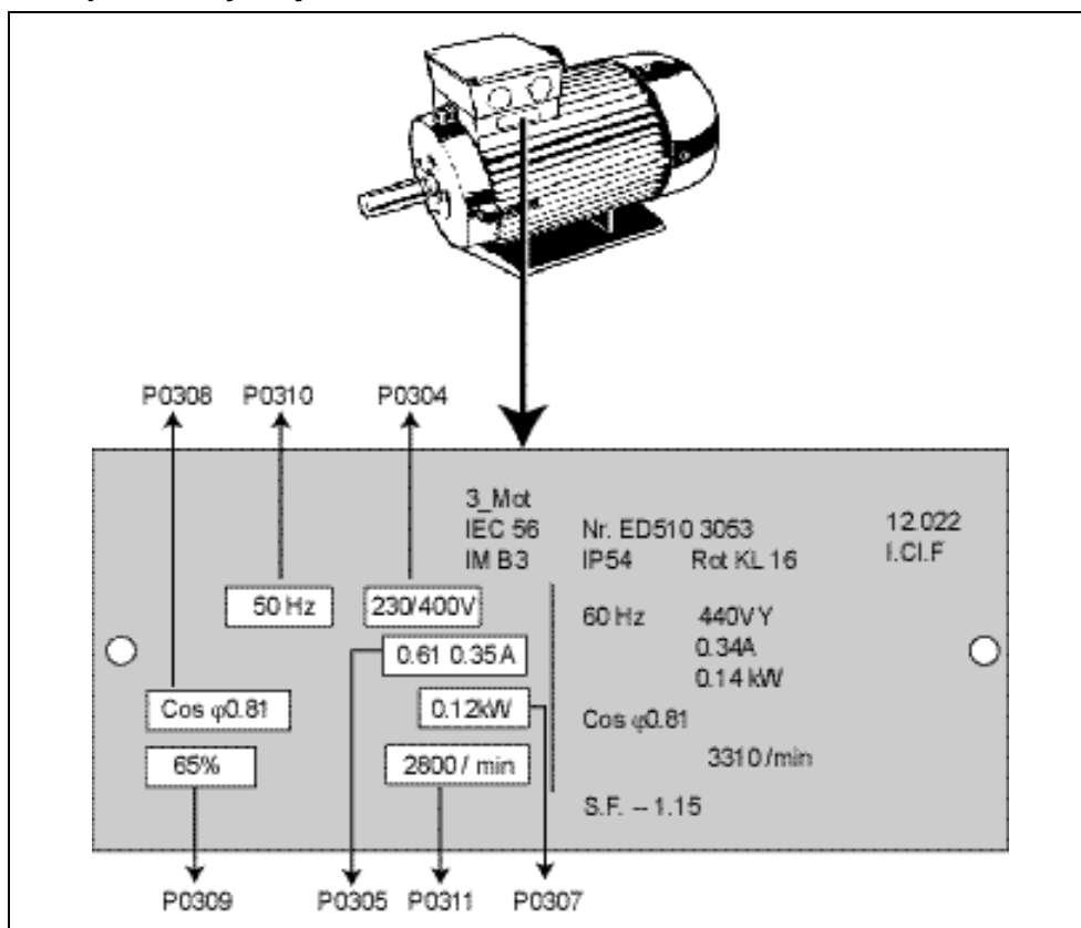
Rys. 3-7 Przykład typowej tabliczki znamionowej silnika (dane na tabliczce znamionowej są tylko przykładowe)
