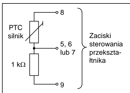
Rys. 3-8 Sposób podłączenia czujnika temperatury uzwojeń silnika
