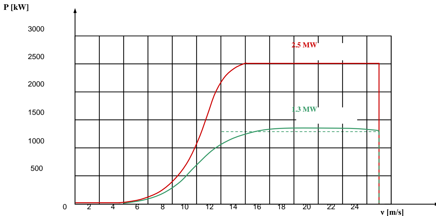
Rys. 2.31. Przykładowe krzywe mocy dla siłowni wiatrowych; Regulacja typu "stall" - 1.3MW (przecignięcie – odpowiednia geometria łopat) Regulacja typu "pitch" - 2.5MW. (zmiana kąta natarcia łopat wirnika)
