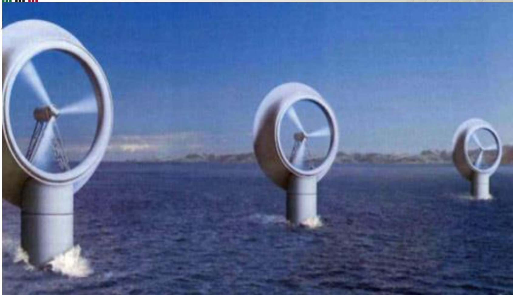
Rys. 44. Turbiny firmy Vortec o średnicy wirnika 66 m i mocy 5 MW.
