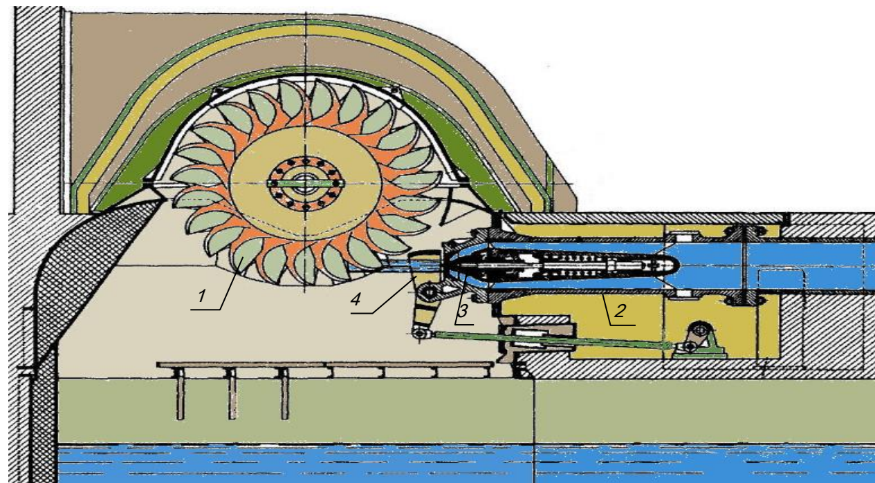
1- łopatka wirnika; 2- dysza; 3- iglica; 4- odchylacz strumienia.
