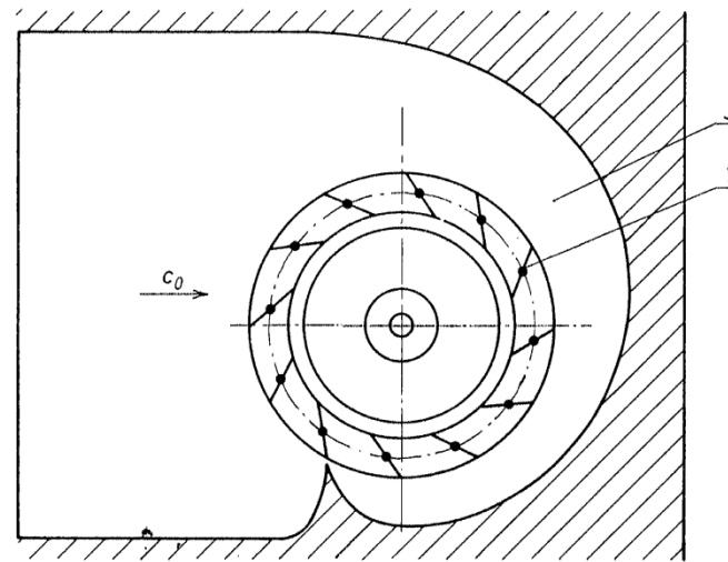
Rys. 12.5. Turbina Kaplana
