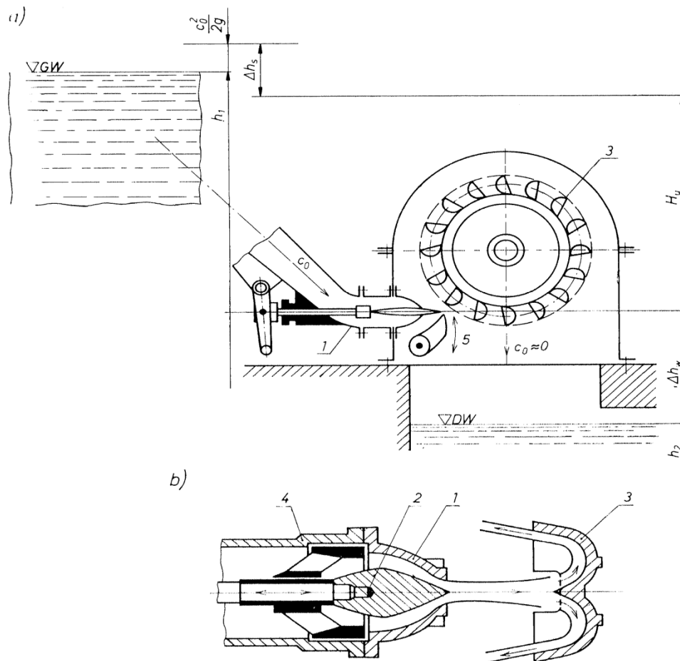
Rys. 12.4. Turbina Peltona: a) doprowadzenie wody i wirnik turbiny; b) dysza i łopatkę wirnika 1 – dysza; 2 – iglica; 3 – łopatkę; 4 – rura ciśnieniowa doprowadzająca wodę; 5 – odchylacz strugi (strumienia); \Delta h_s – straty spadujące przy przepływie wody przez utorociąg, budowle i urządzenia
