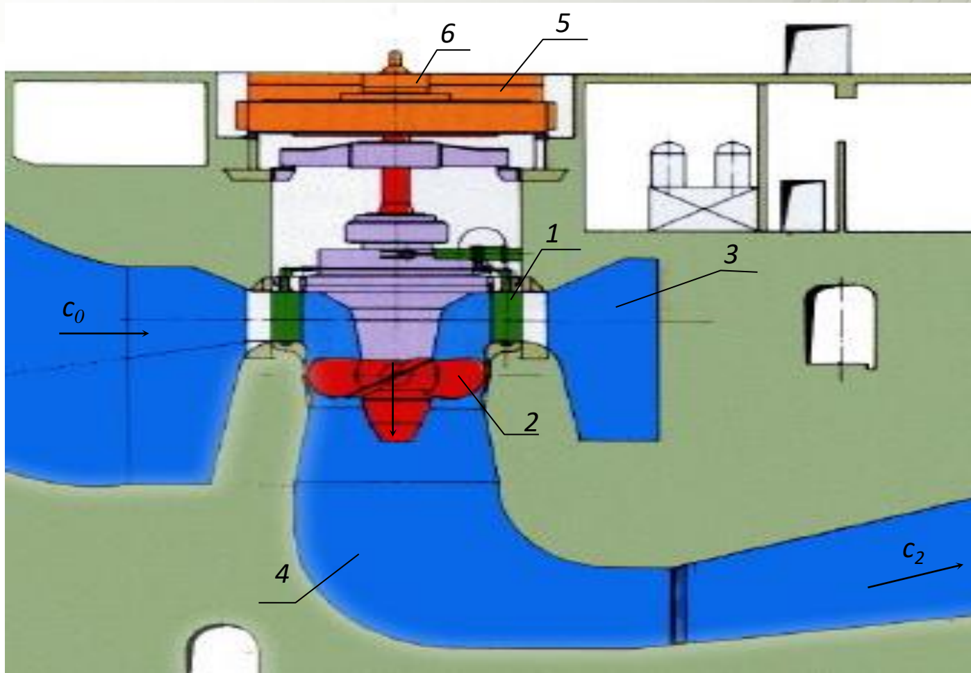
Przekrój elektrowni wykorzystującej turbinę Kaplana: 1 - łopatki kierownicze; 2 - łopatki wirnika; 3 - spirala doprowadzająca wodę (betonowa); 4 - rura ssąca; 5 - generator; 6 - wzбудnica
