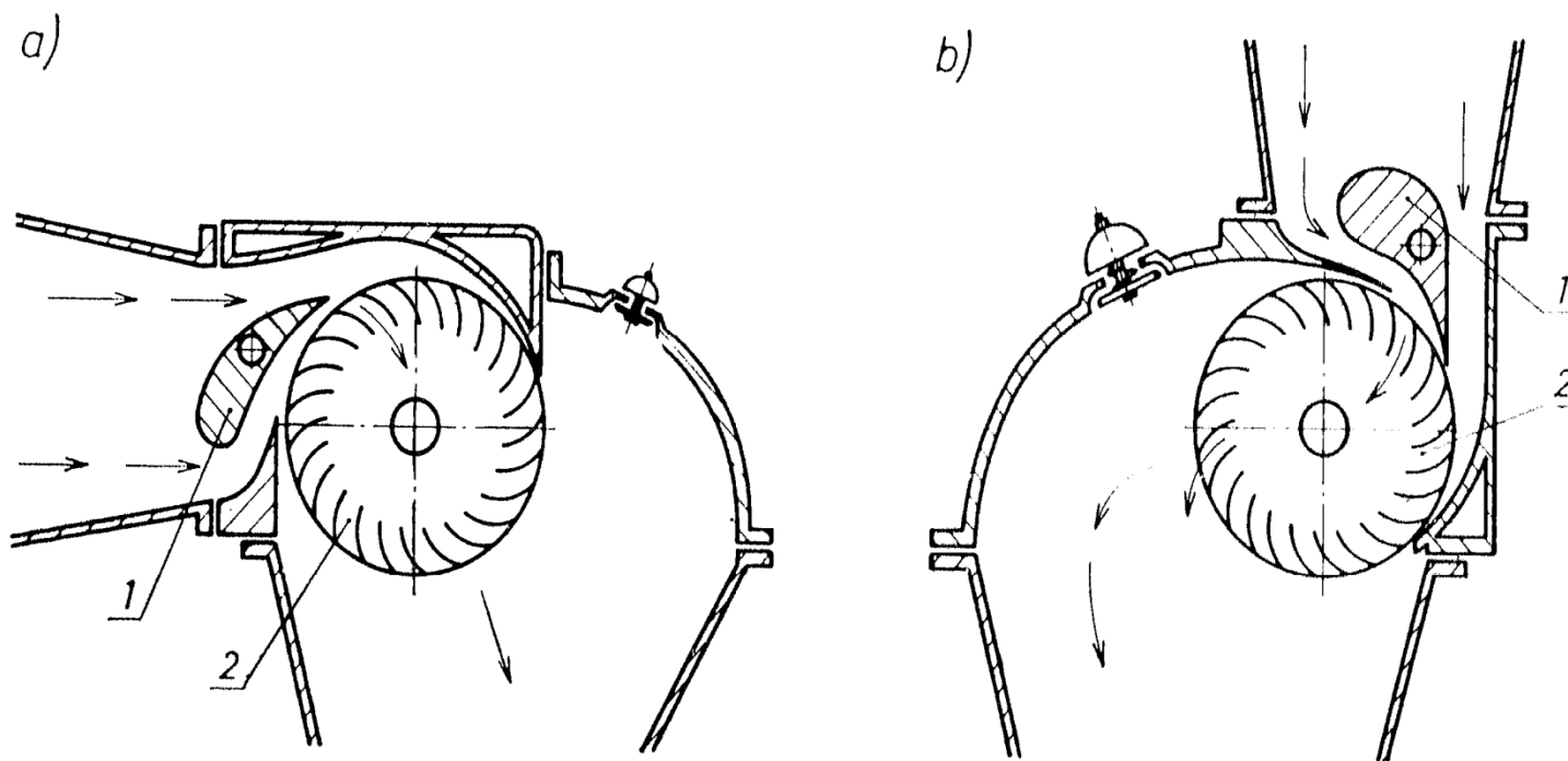
Rys. 12.10. Turbina Banki-Michella z napływem: a) poziomym; b) pionowym wg materiałów informacyjnych firmy Ossberger-Turbinenfabrik Weissenburg RFN
