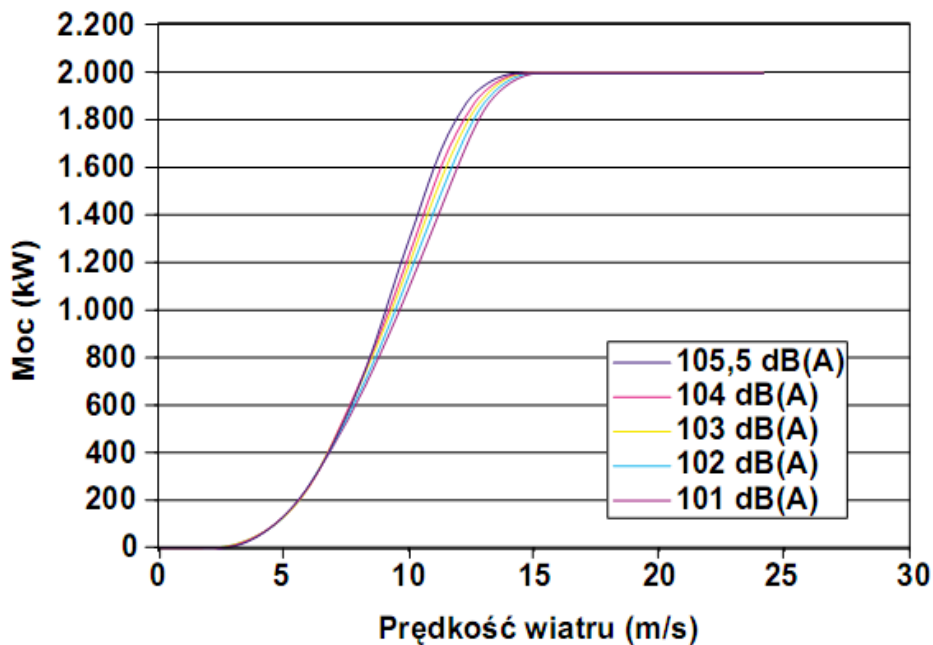
Krzywa mocy modelu V80-2,0 MW
