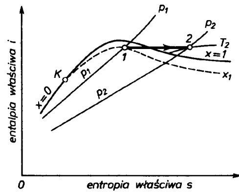
dławienie izentalpowe (i=idem):
