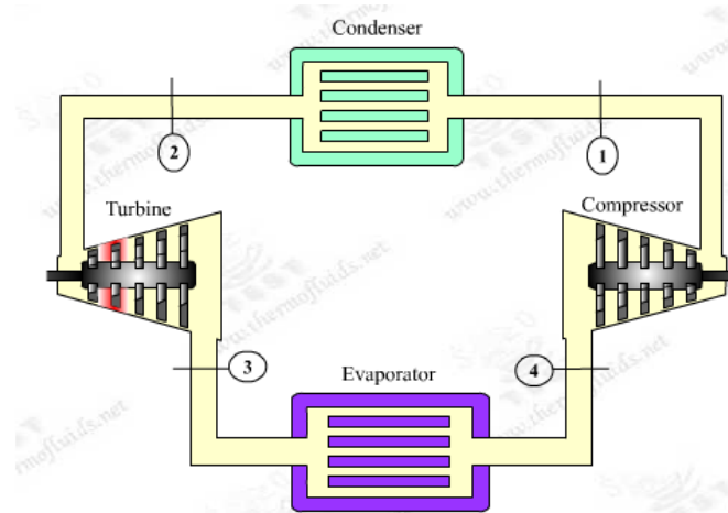
Rys.4. Układ chłodniczy realizujący obieg Joule'a
