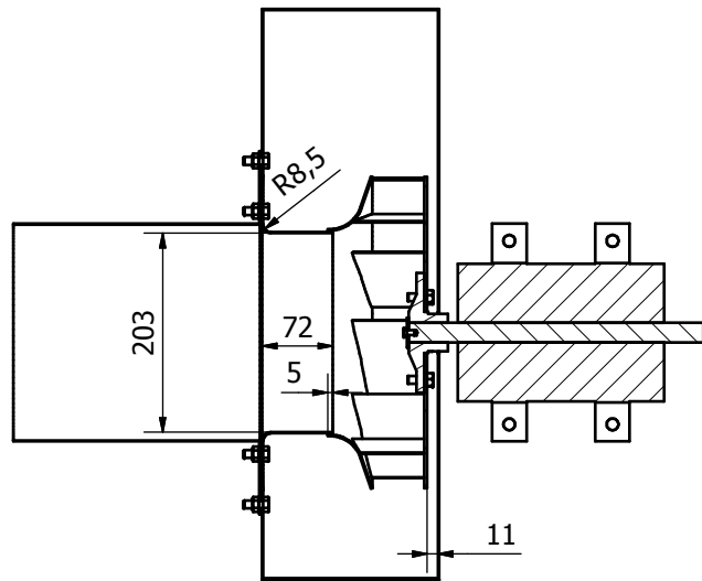
A-A ( 1:6 )
