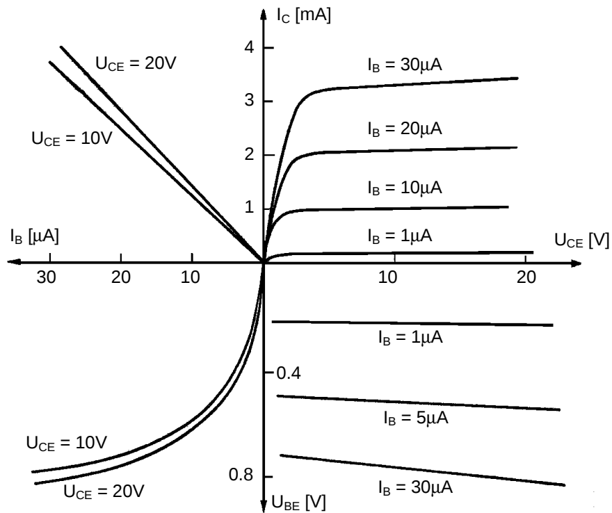
charakterystyki tranzystora bipolarnego (wspólny emiter)
