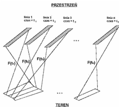
Rys.1 Schematyczny rysunek przedstawiający sposób działania sensora skanującego. Poszczególne linijki detektorów, rejestrują odpowiadające im pasy pokrycia terenu [8].
